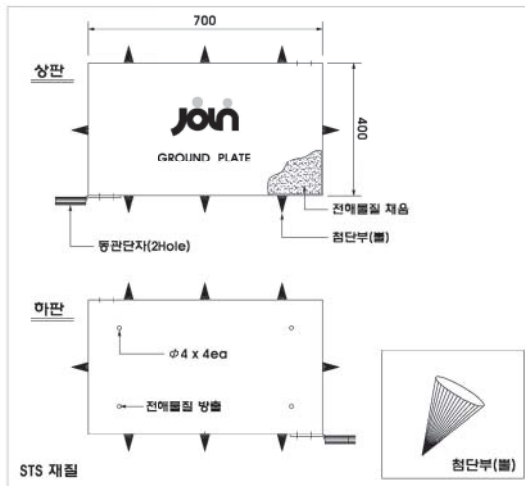
STS 전해질 방사형 접지판 (GP-700) 상세도
