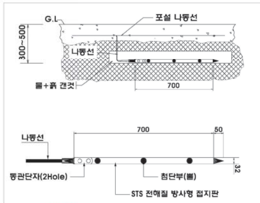
STS 전해질 방사형 접지판 (GP-700) 설치 상세도
